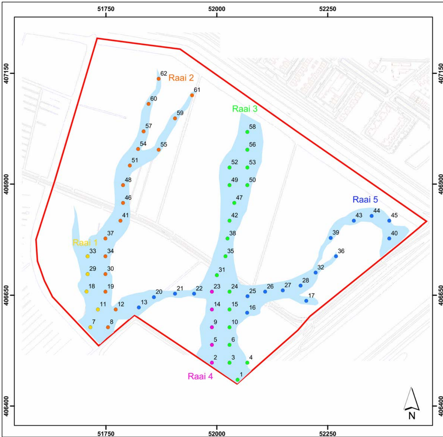
Afbeelding 9. De Boorpuntenkaart van het IVO-Overig, geprojecteerd op een uitsnede van de GBKN, met Boorraai 1 t/m 5. Bron: Van den Bosch, 2013a. Schaal 1: 5.000.
