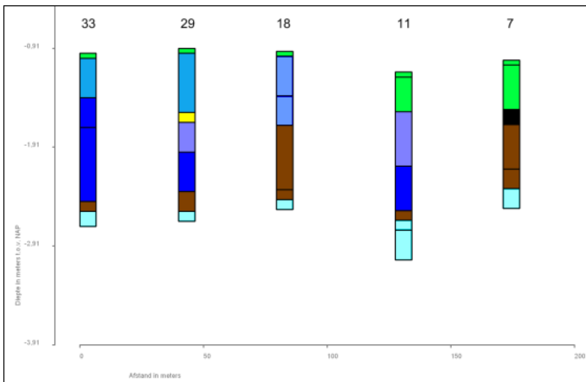
Afbeelding 10. De dwarsprofielen van Boorraai 1 (IVO-Overig). Bron: Van den Bosch, 2013a.
