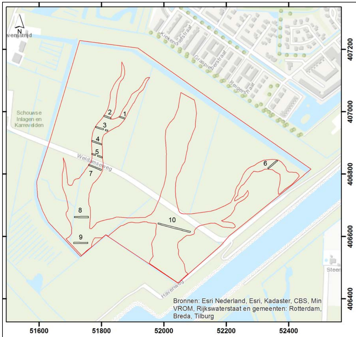
Afbeelding 17. De overzichtskaart met de tijdens het IVO-P aangelegde proefsleuven (zwart omkaderd en genummerd), ter plaatse van de geplande krekens. Schaal 1: 7.500.
