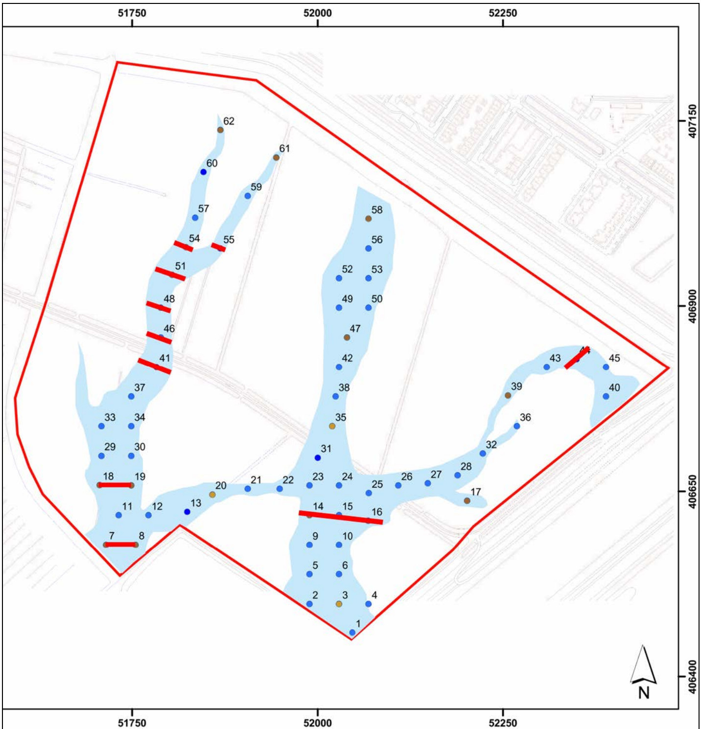
Afbeelding 8. De boorpuntenkaart van het IVO-Overig, met daarop geprojecteerd de binnen het onderzoeksgebied aan te leggen proefsleuven (rood gemarkeerd). Bron: Programma van Eisen; Van den Bosch, 2013b. Schaal 1: 5.000.
