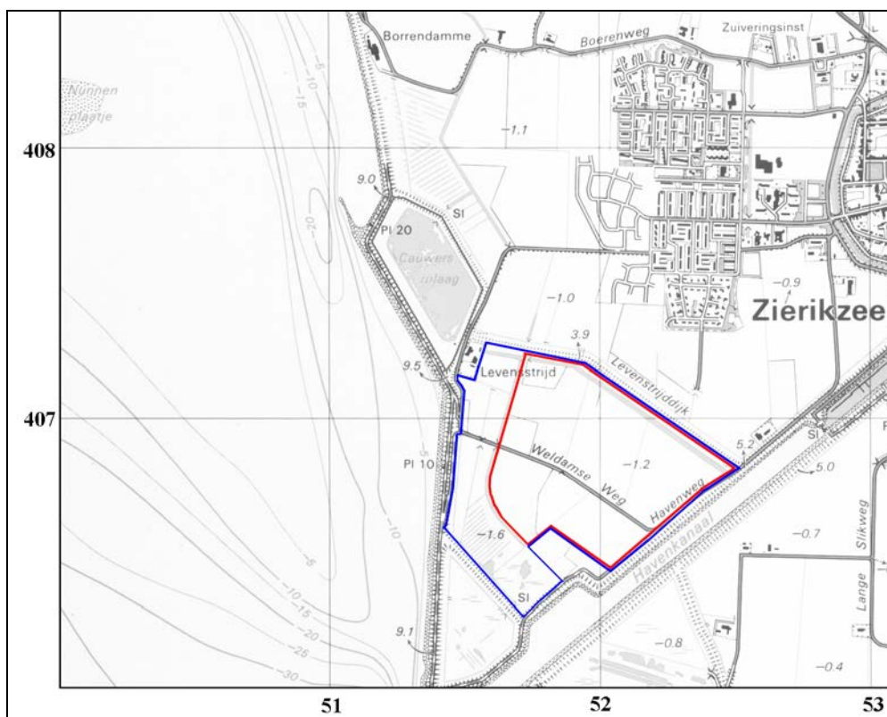
Afbeelding 3. De ligging van het plangebied (blauw omkaderd), geprojecteerd op een uitsnede van de Topografische Kaart. De globale zone waarbinnen het onderzoeksgebied van het IVO-Overig was gelegen is rood omkaderd. Bron: Van den Bosch, 2013a. Schaal 1: 25.000.
